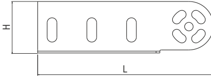
60/75/100 CT-SDE L=160
